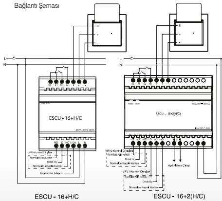
Bağlantı Şeması
