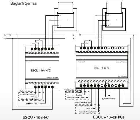
Bağlantı Şeması
